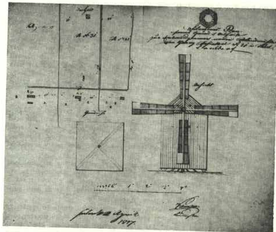
Plán ke stavbě větráku ve Vrchách č. 31 z roku 1847
